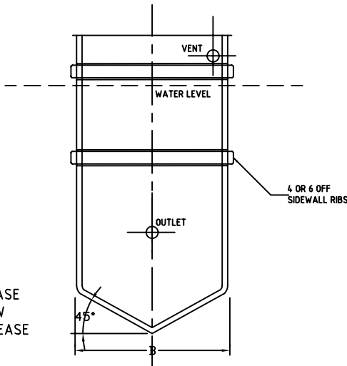
END ELEVATION
